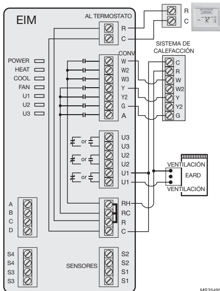
Fig. 3. Cómo cablear un EARD a un VisionPRO® con RedLINK™.
