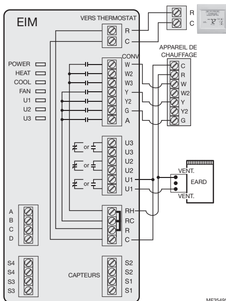
Fig. 3. Câblage du modèle EARD à un VisionPRO® avec RedLINK™.
