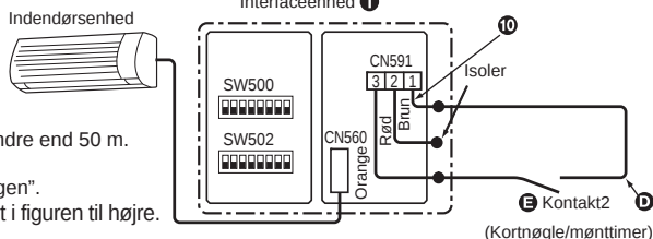
Forbindelse af kortnøgle og mønttimer
