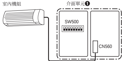
使用電源開 / 關功能時的設定
