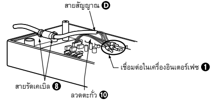
การเชื่อมต่อคีย์การ์ดและตัวตั้งเวลา
