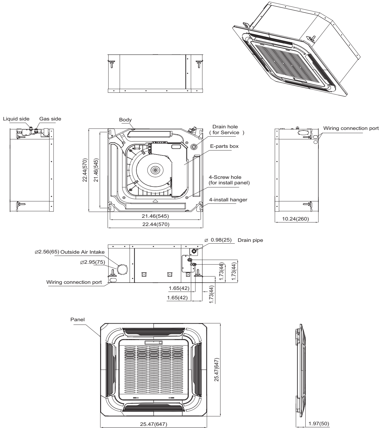
Fig. 1 – Indoor Unit
