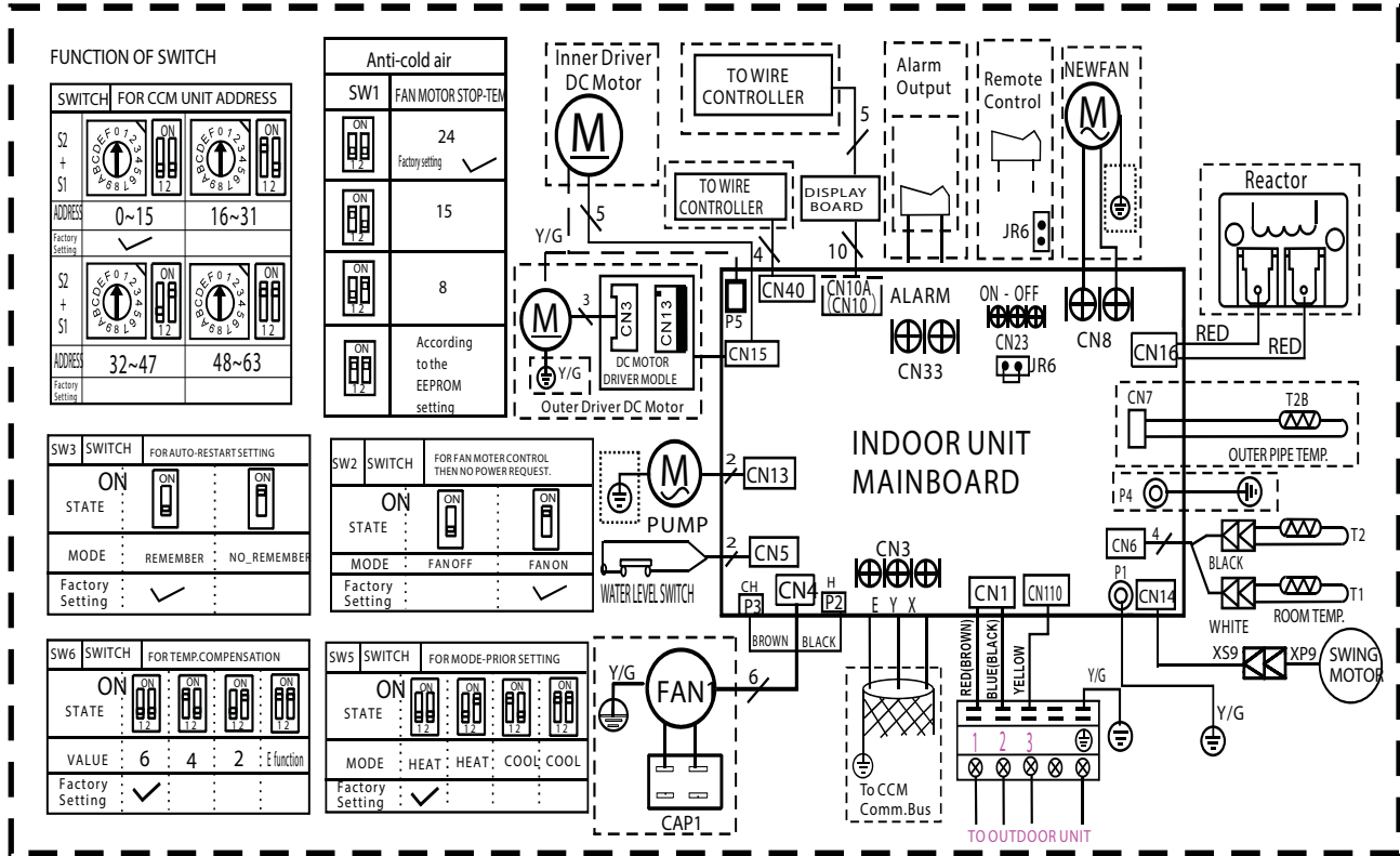
Fig. 7 – Wiring Diagram
