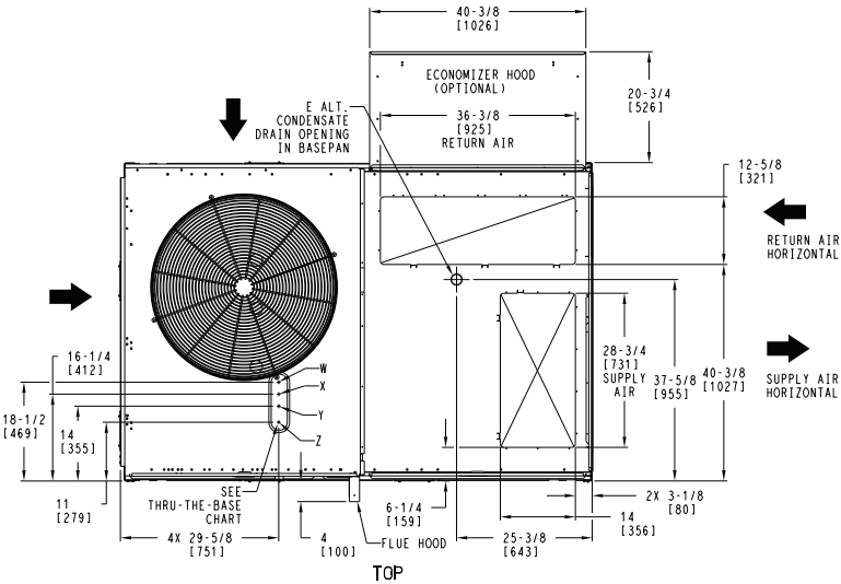
TOP
