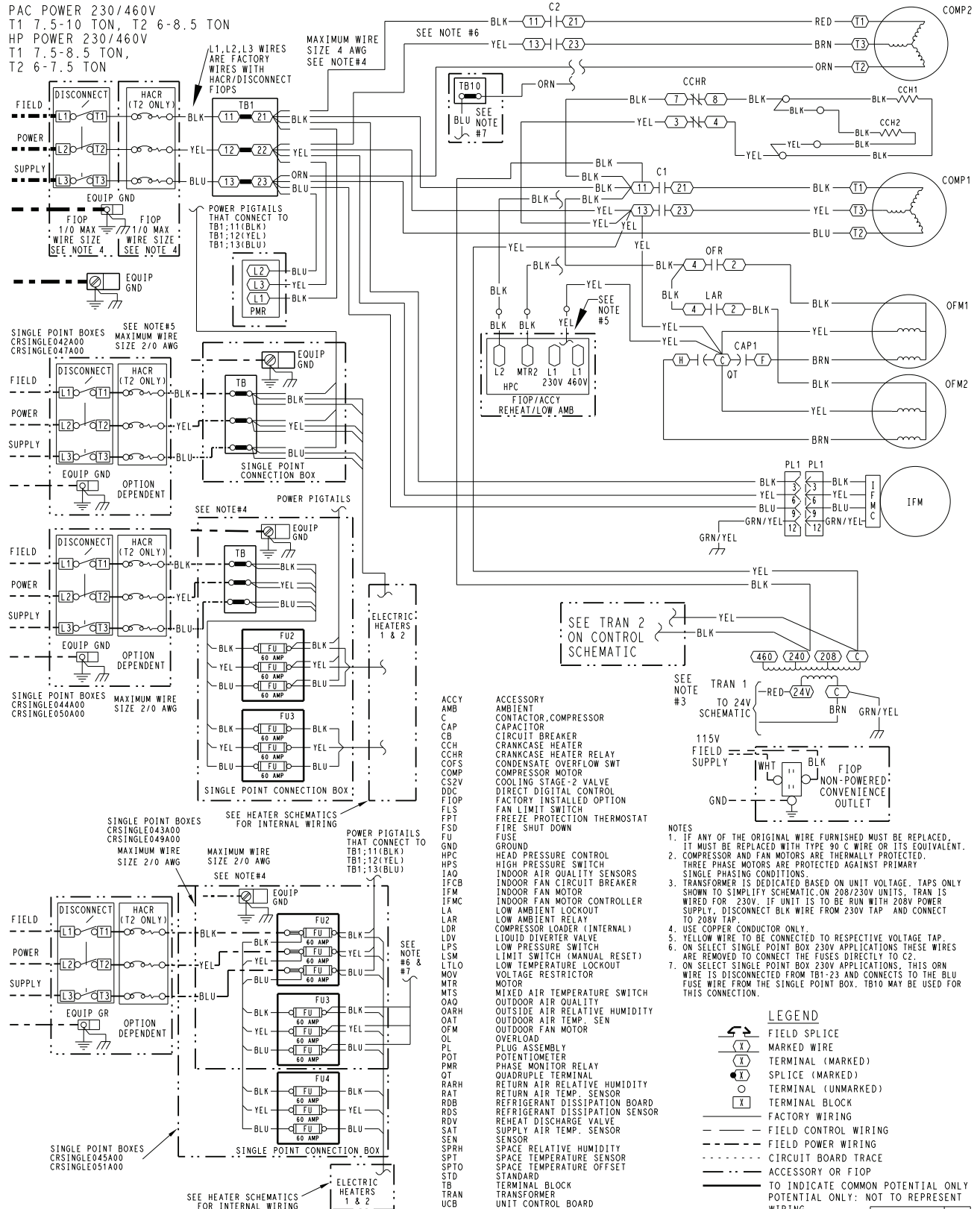
RHF090-102 Power Wiring Diagram, 230/460-3-60 Shown
